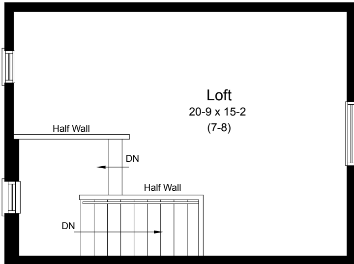
Optional Loft Floor Plan 362 sq.ft.
