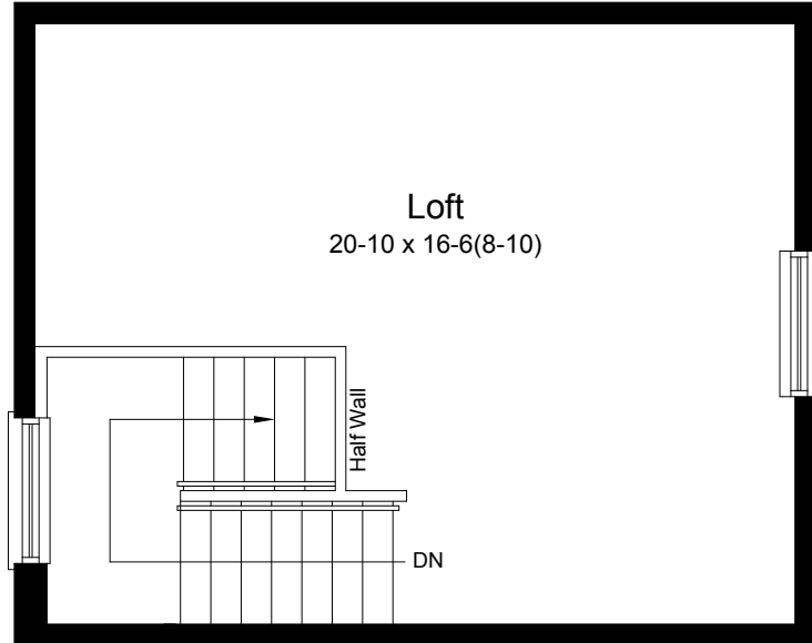
Optional Loft Floor Plan 388 sq.ft.
